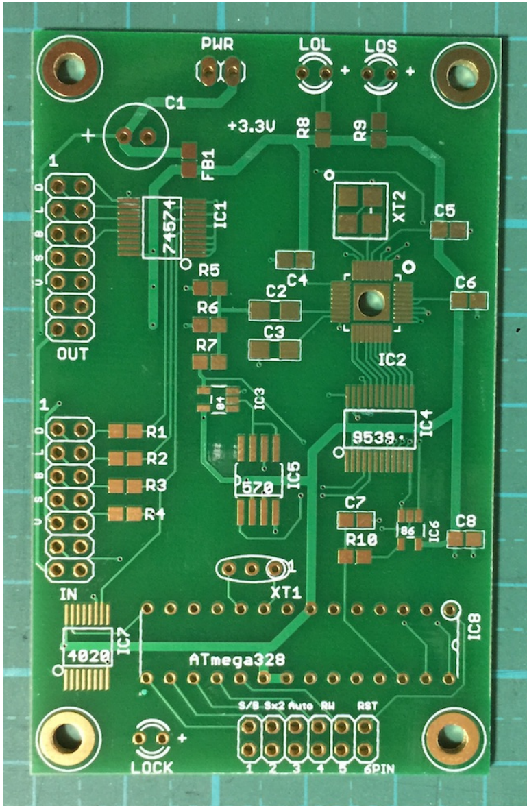
リニューアル版I2Sリクロック基板の裏面
