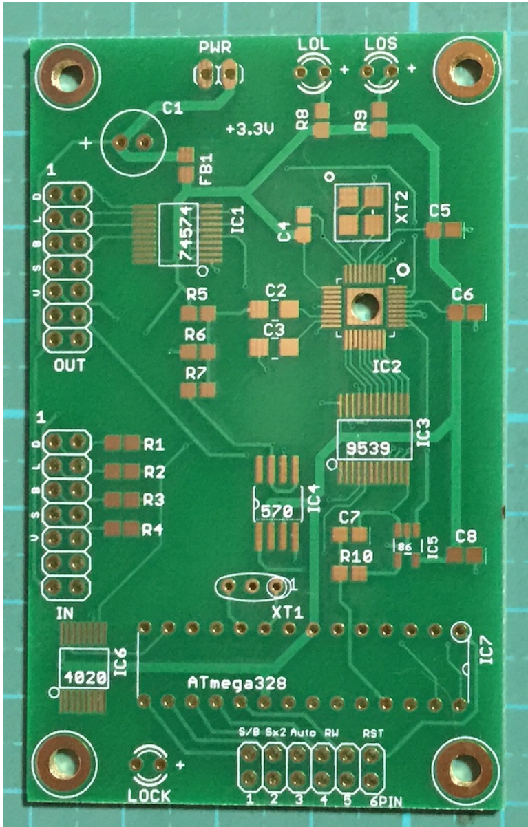
I2Sリクロック基板の裏面
