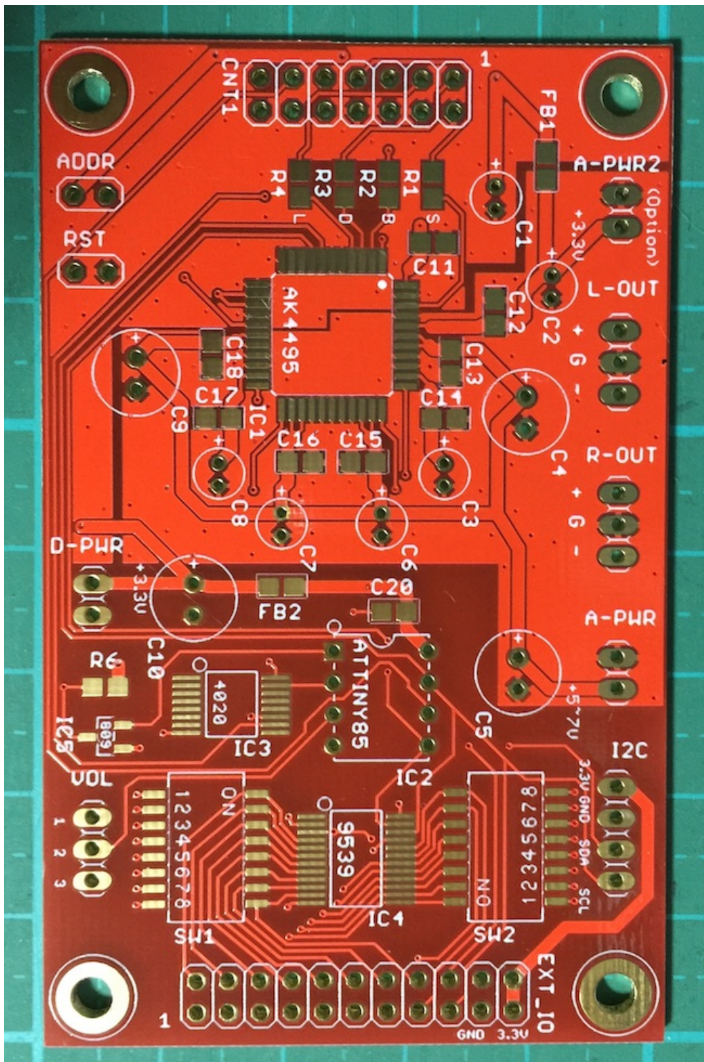
AK4495S DAC基板の裏面
