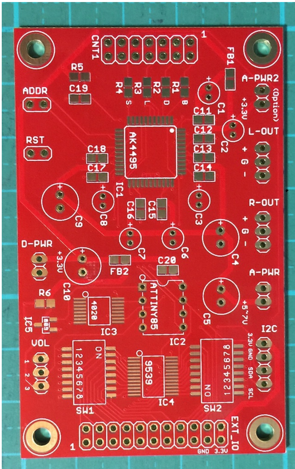
AK4495S DAC基板の裏面
